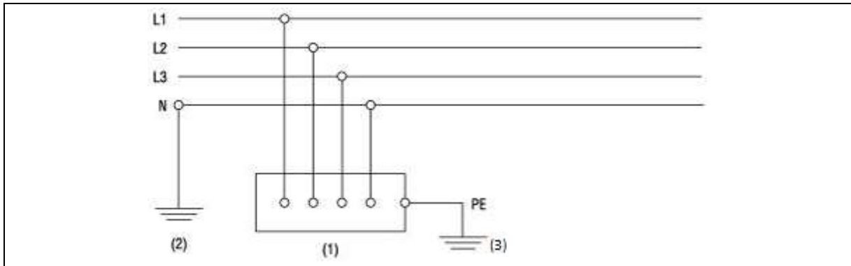
Figure 3.4. Schéma TT
