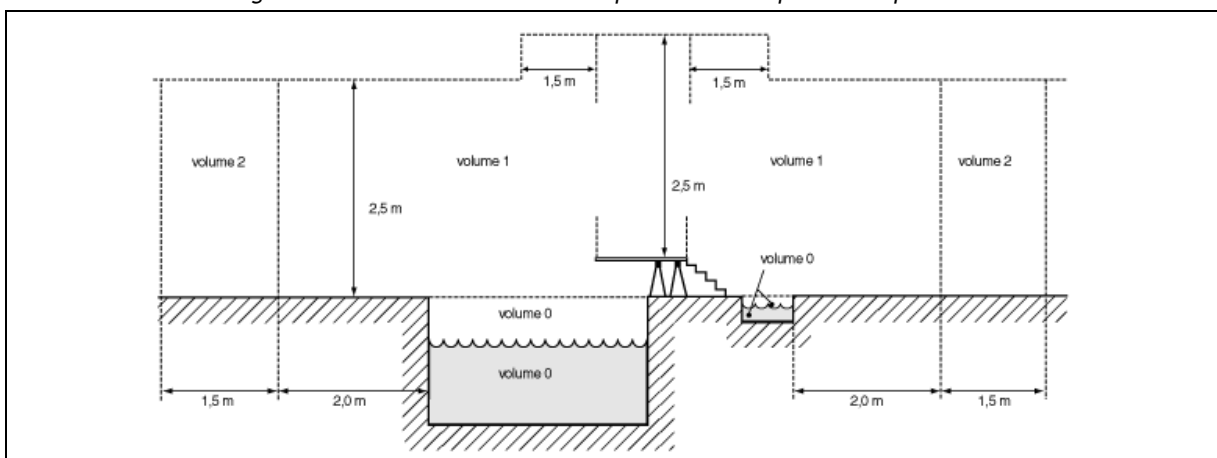
Figure 7.12. Dimensions des volumes pour bassins de piscines et pédiluves
